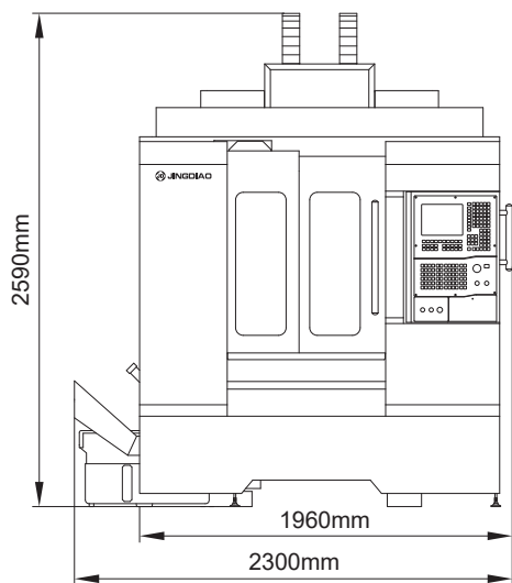
前视图
