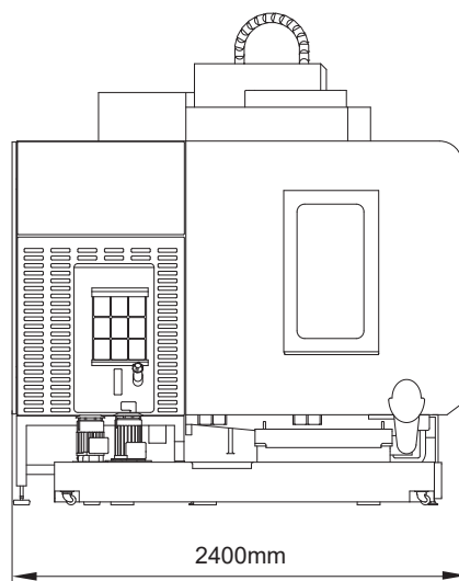
左视图
