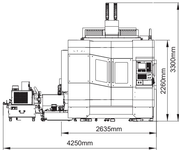
前视图
