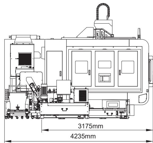
左视图
