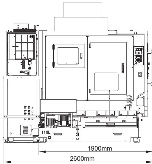
左视图
