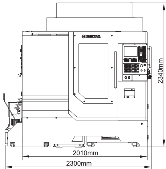
前视图
