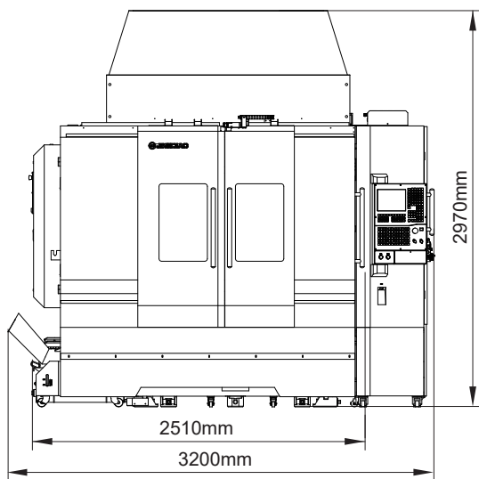
前视图
