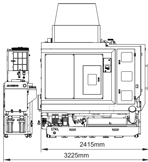
左视图
