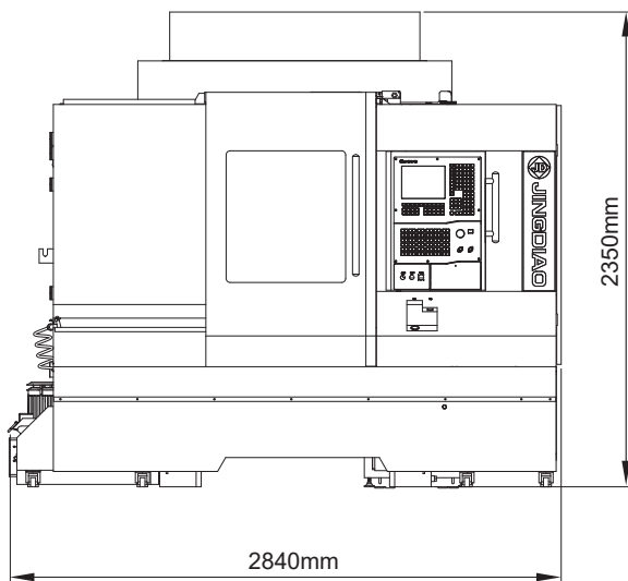
前视图
