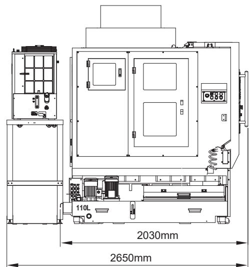
左视图
